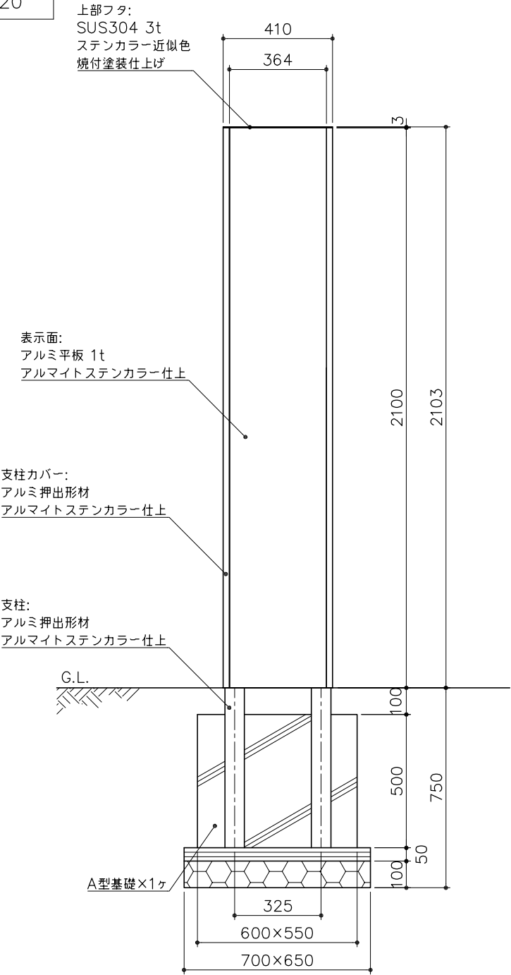
立面図 S= 1:20
