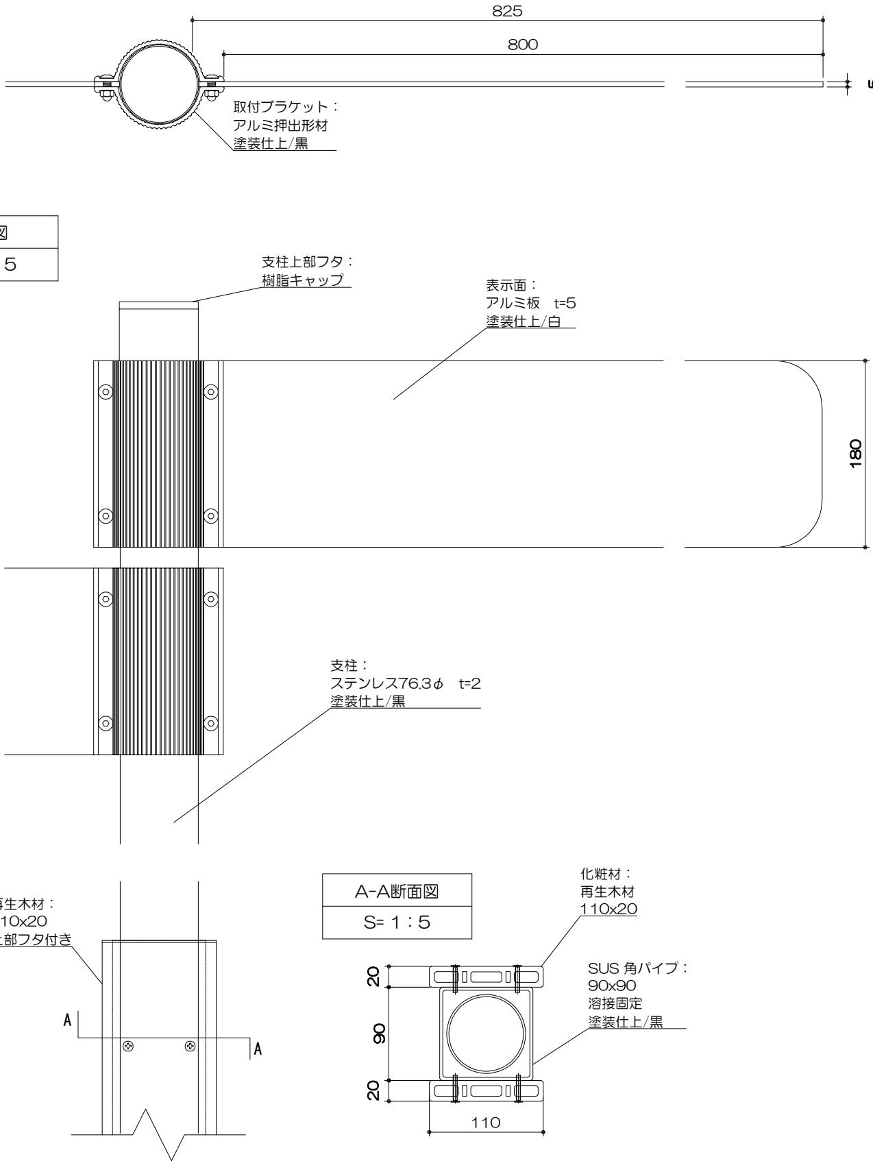
平面図 S= 1 : 5
