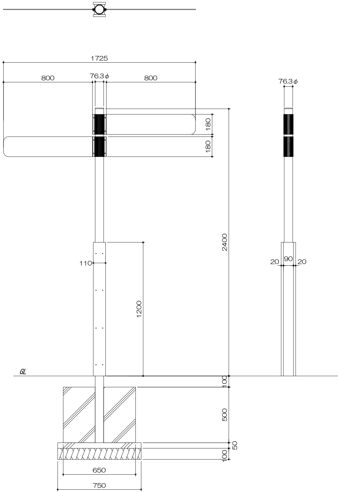
正面図 S= 1 : 5
