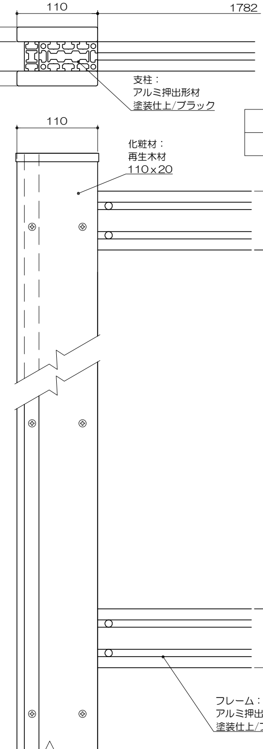
立面図 S= 1 : 5
