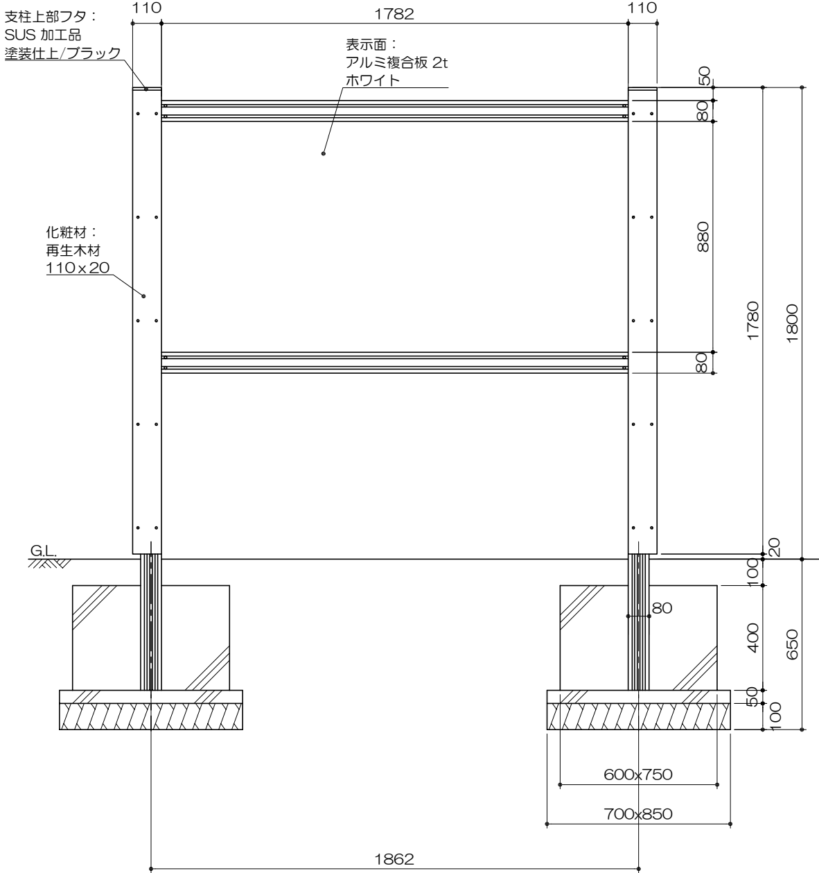
立面図 S= 1 : 20
