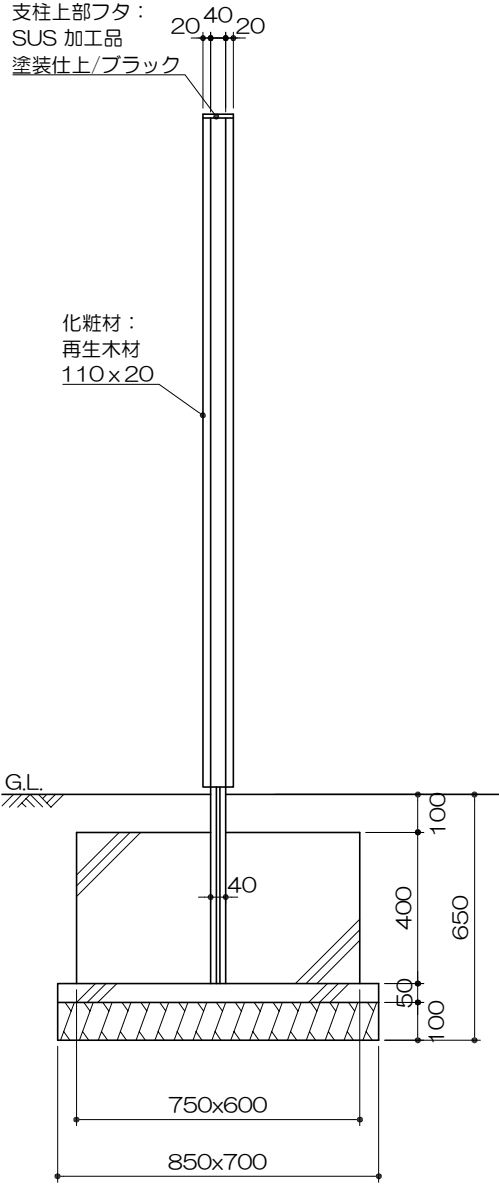
側面図 S= 1 : 20
