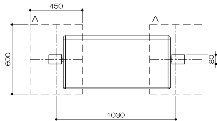
立面図 S= 1 : 20
