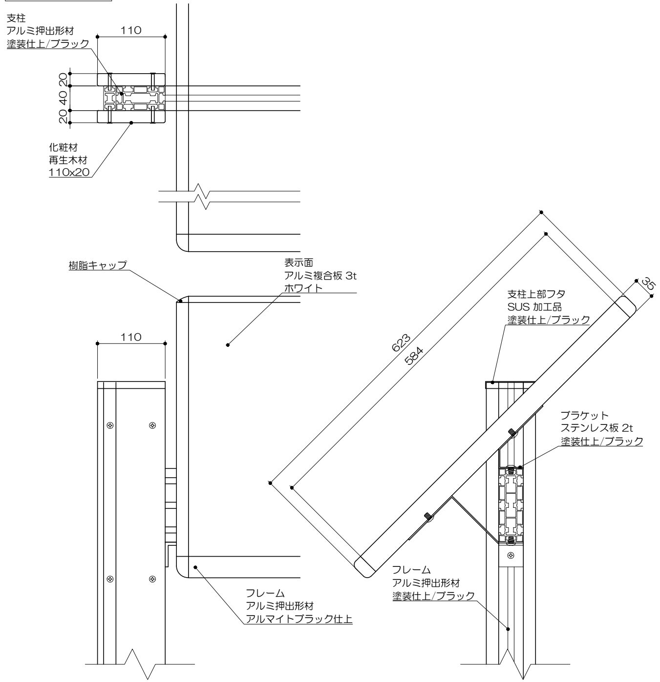
詳細図 S= 1 : 6
