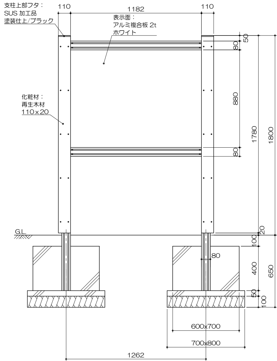
立面図 S= 1 : 20
