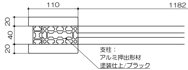
断面図 S= 1 : 5
