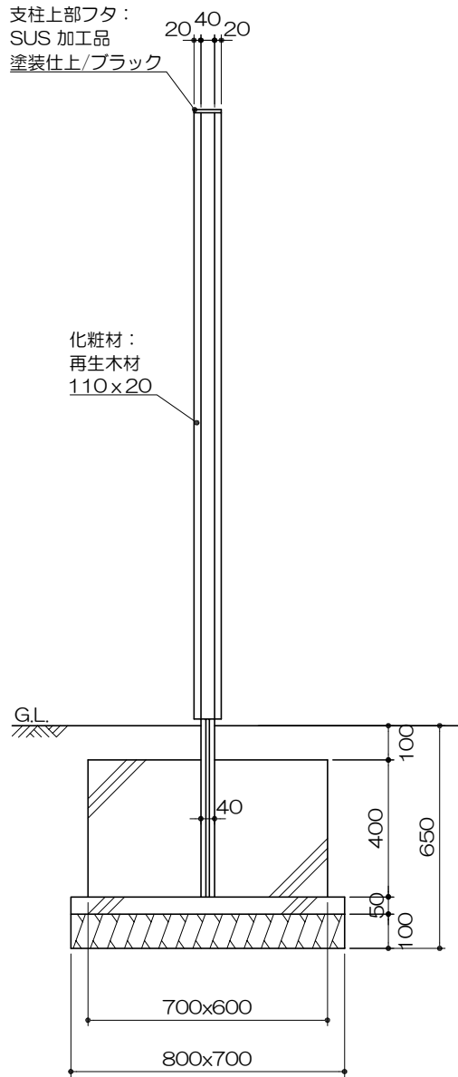
正面図 S= 1 : 5
