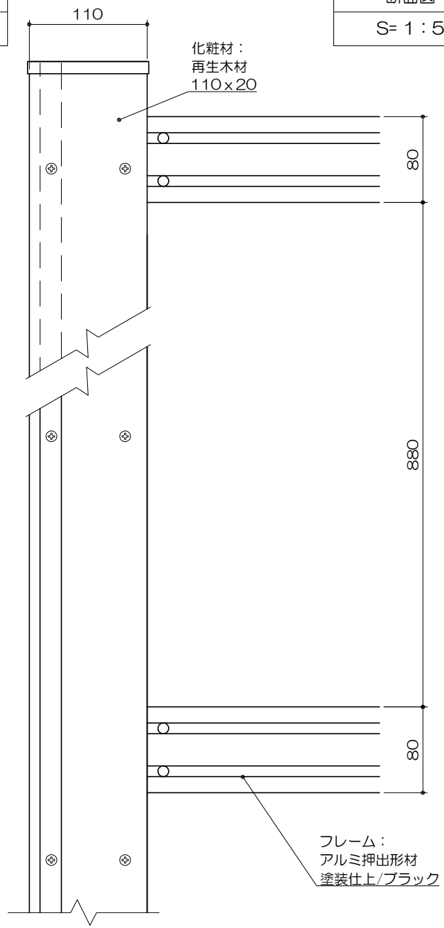
正面図 S= 1 : 5
