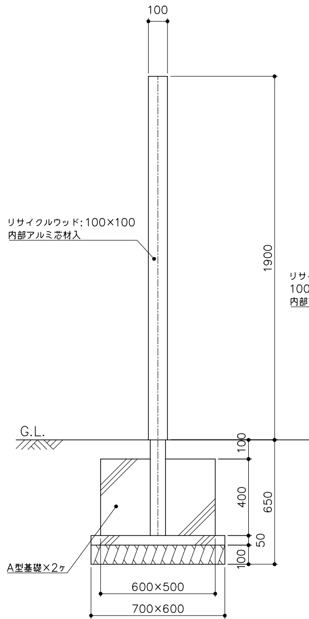
側面図 S= 1 : 20
