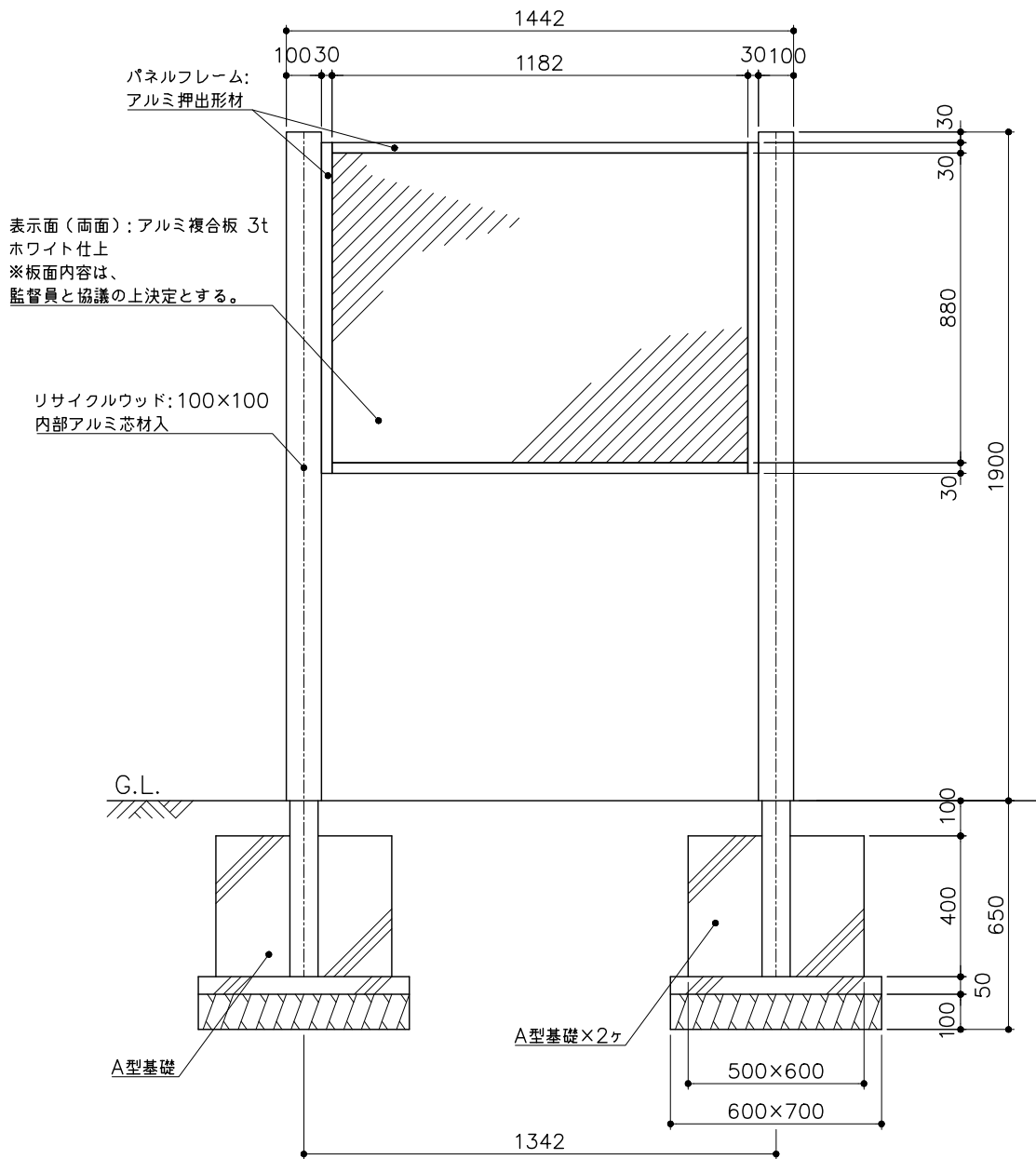
立面図 S= 1 : 20
