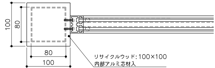
正面図 S= 1 : 5
