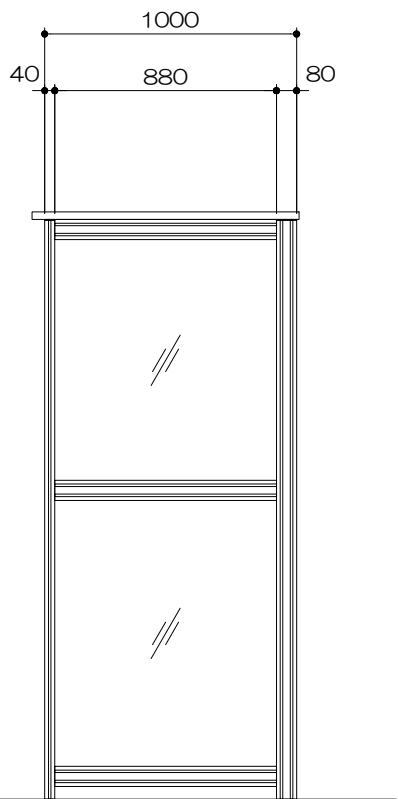
側面図 S= 1 : 30
