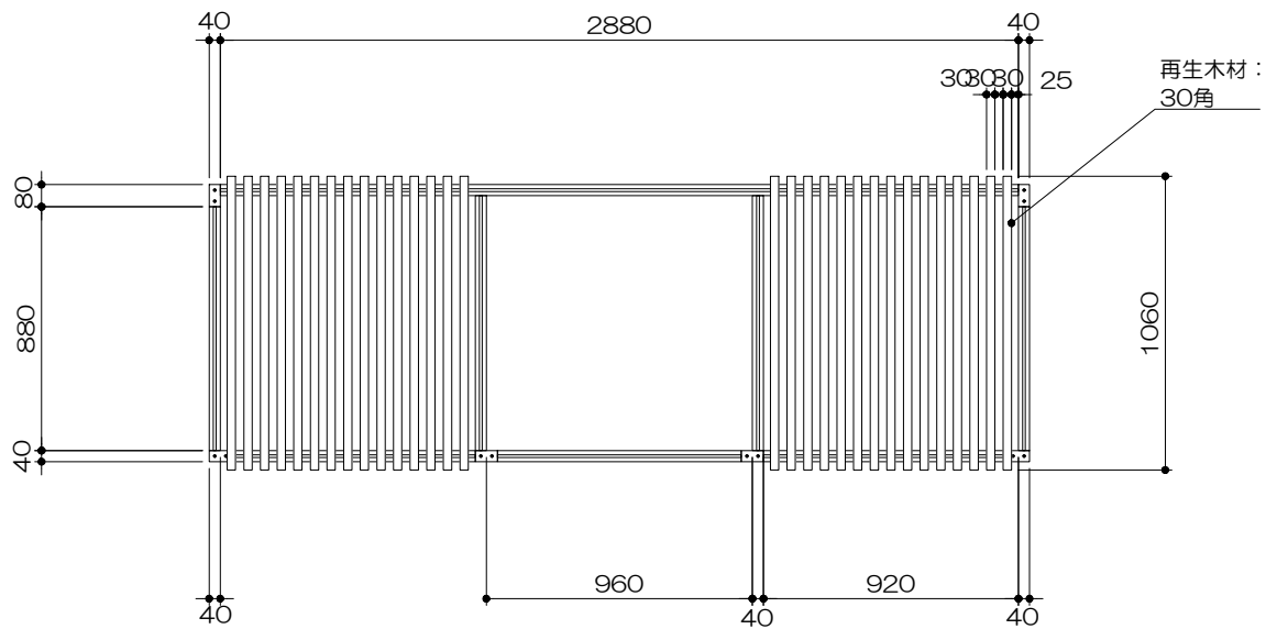
平面図 S= 1 : 30
