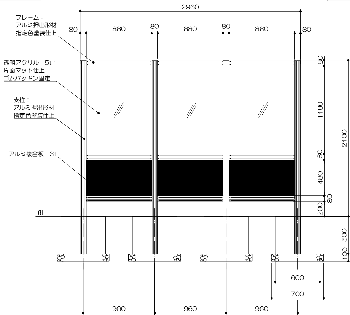
正面図 S= 1 : 30
