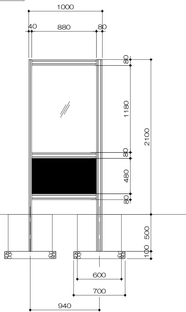
側面図 S= 1 : 30
