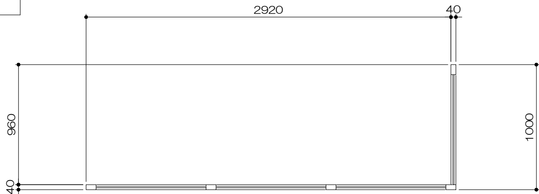
側面図 S= 1 : 30
