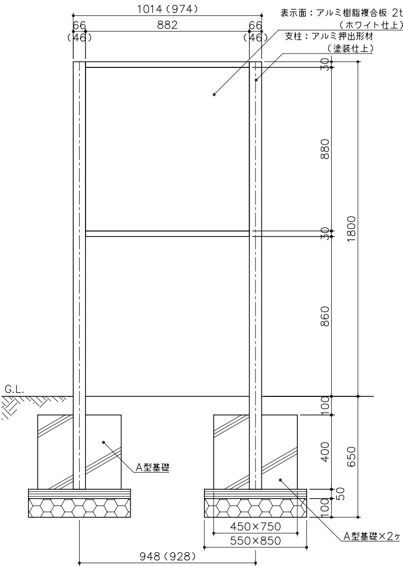
立面図 S= 1：20
