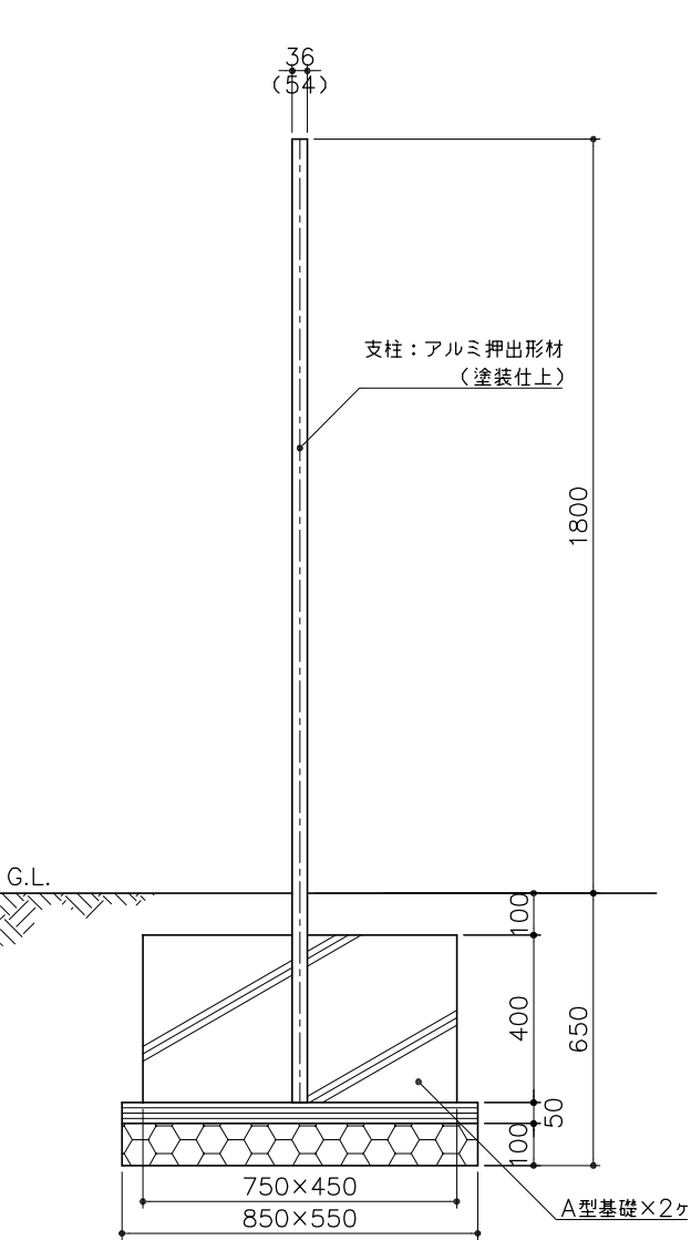
立面図 S= 1：3
