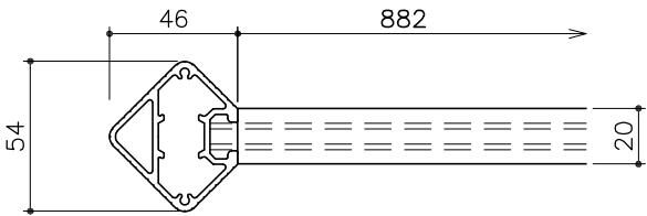
平面図 S= 1：3
