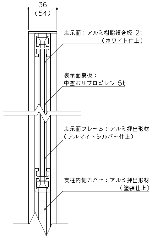
断面図 S= 1：3
