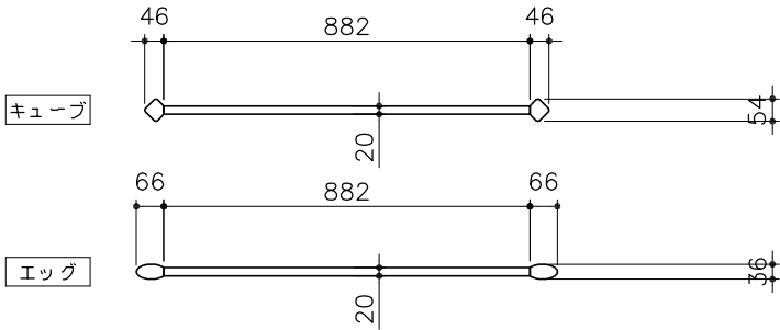
平面図 S= 1：20
