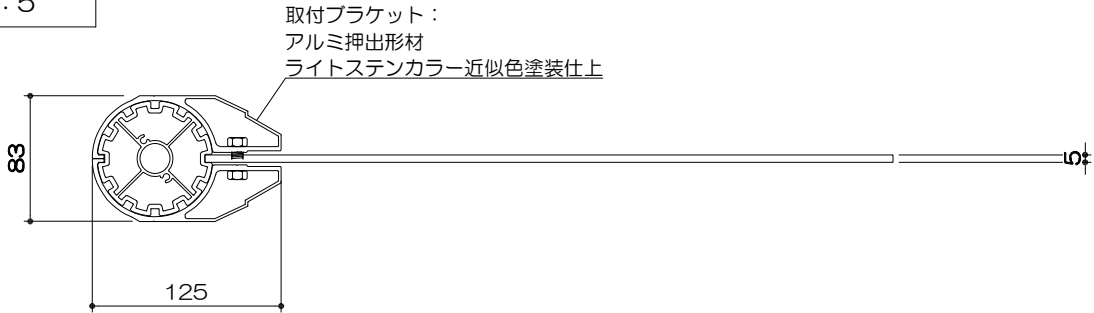
平面図 S= 1 : 5
