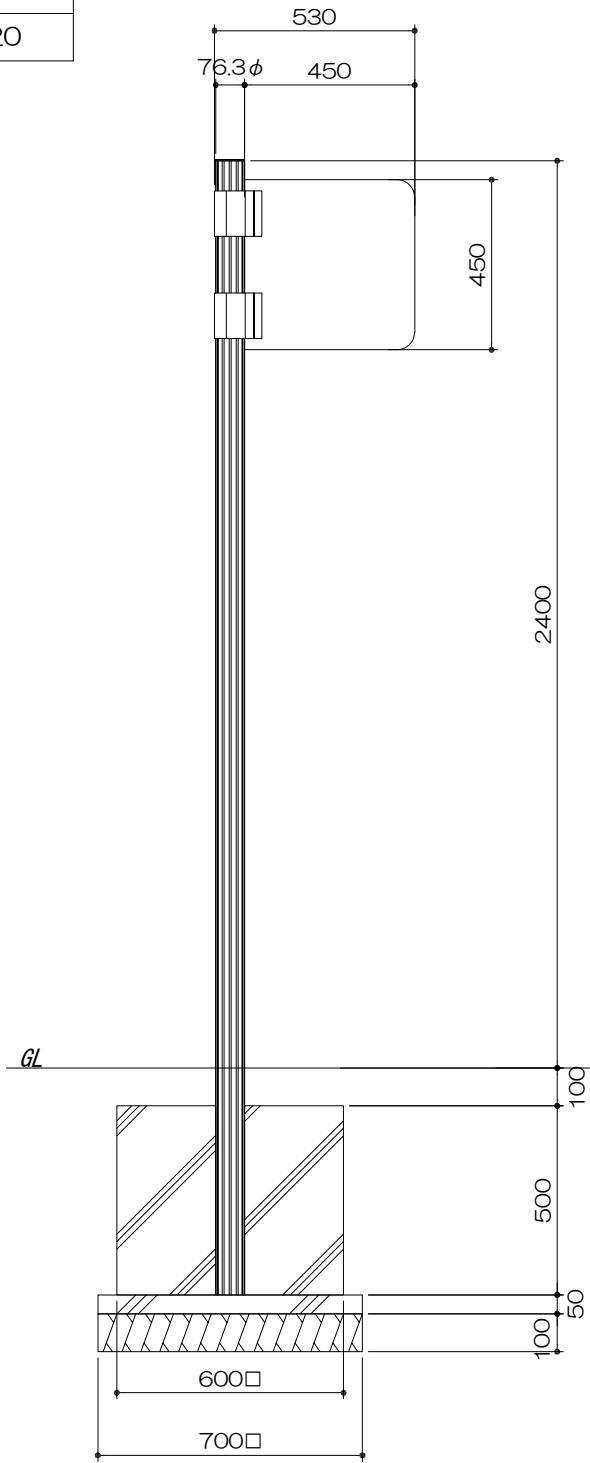
側面図 S= 1 : 20
