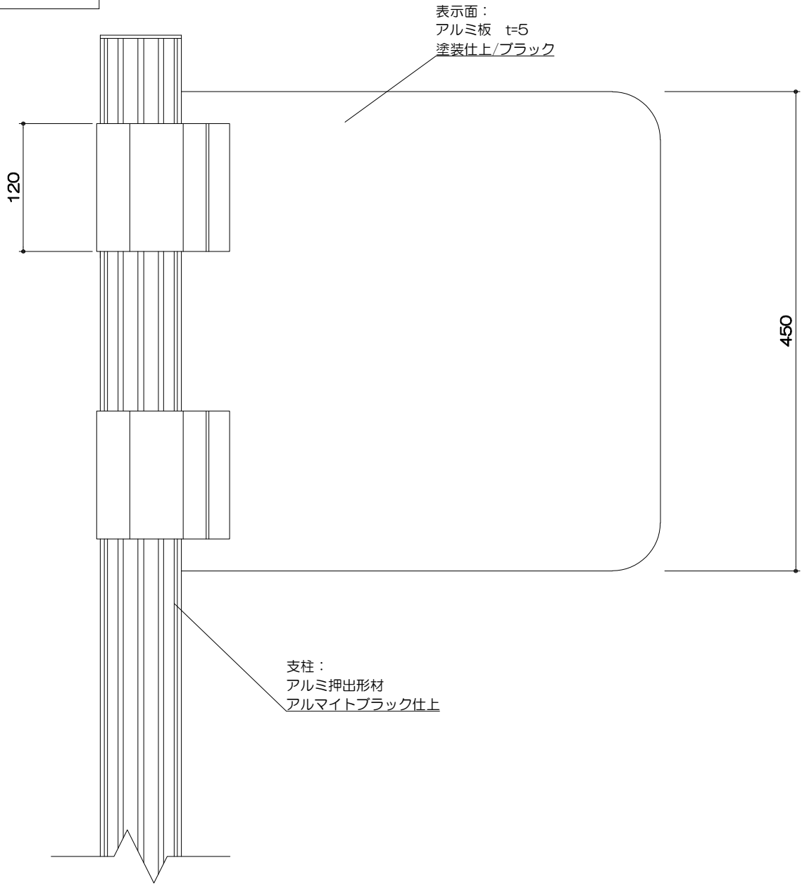
正面図 S= 1 : 5
