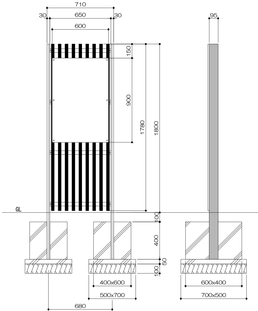
正面図 S= 1 : 20
