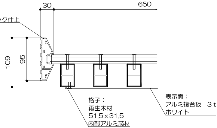
平面図 S= 1 : 5
