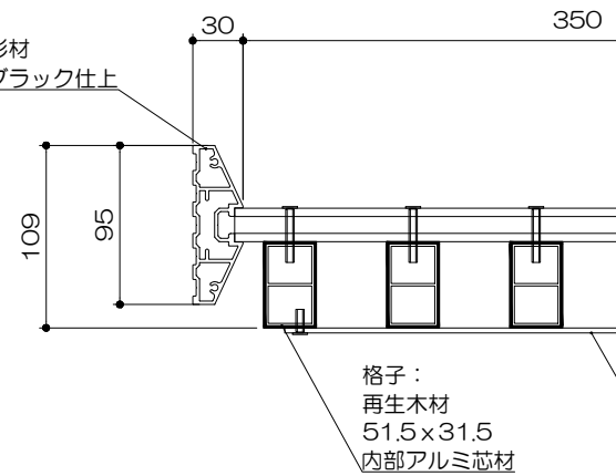
立面図 S= 1 : 5
