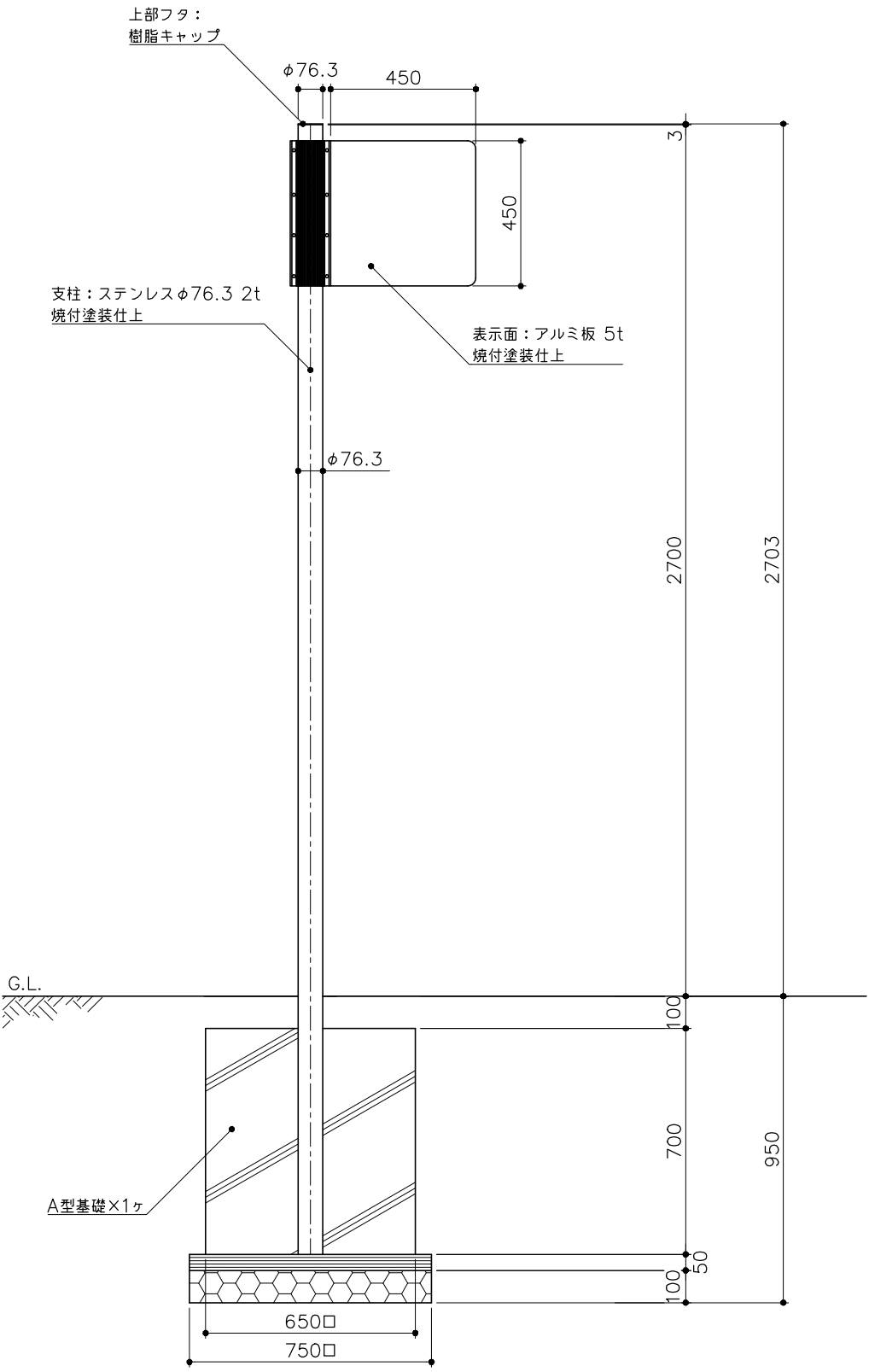
立面図 S= 1:20
