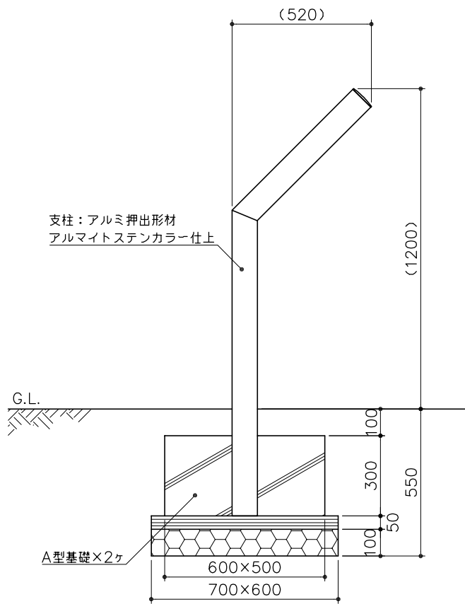
側面図 S= 1：20
