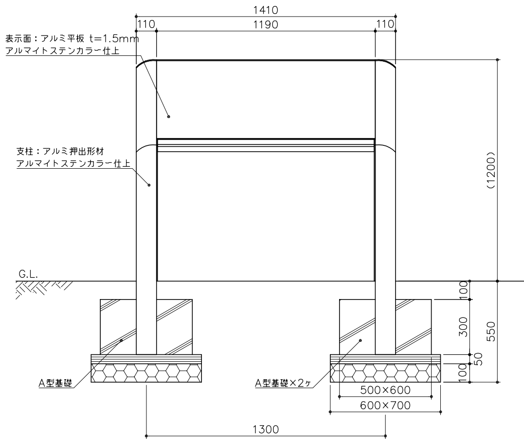
立面図 S= 1：20
