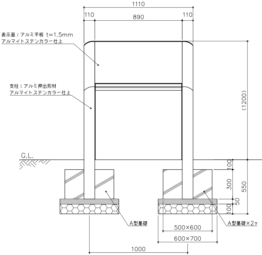
立面図 S= 1：20
