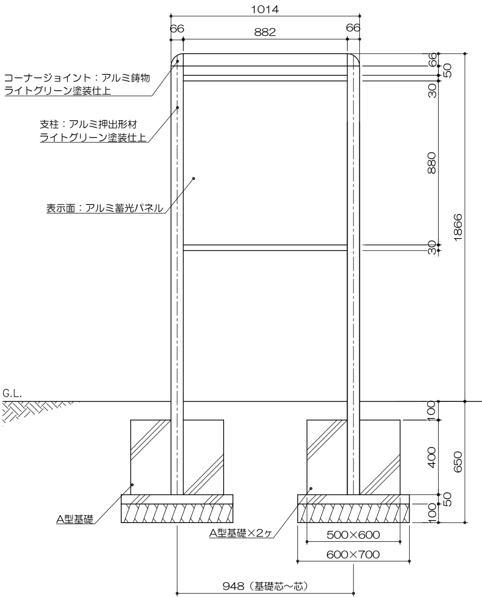
立面図 S= 1:20
