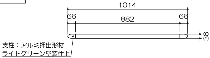
平面図 S= 1:20
