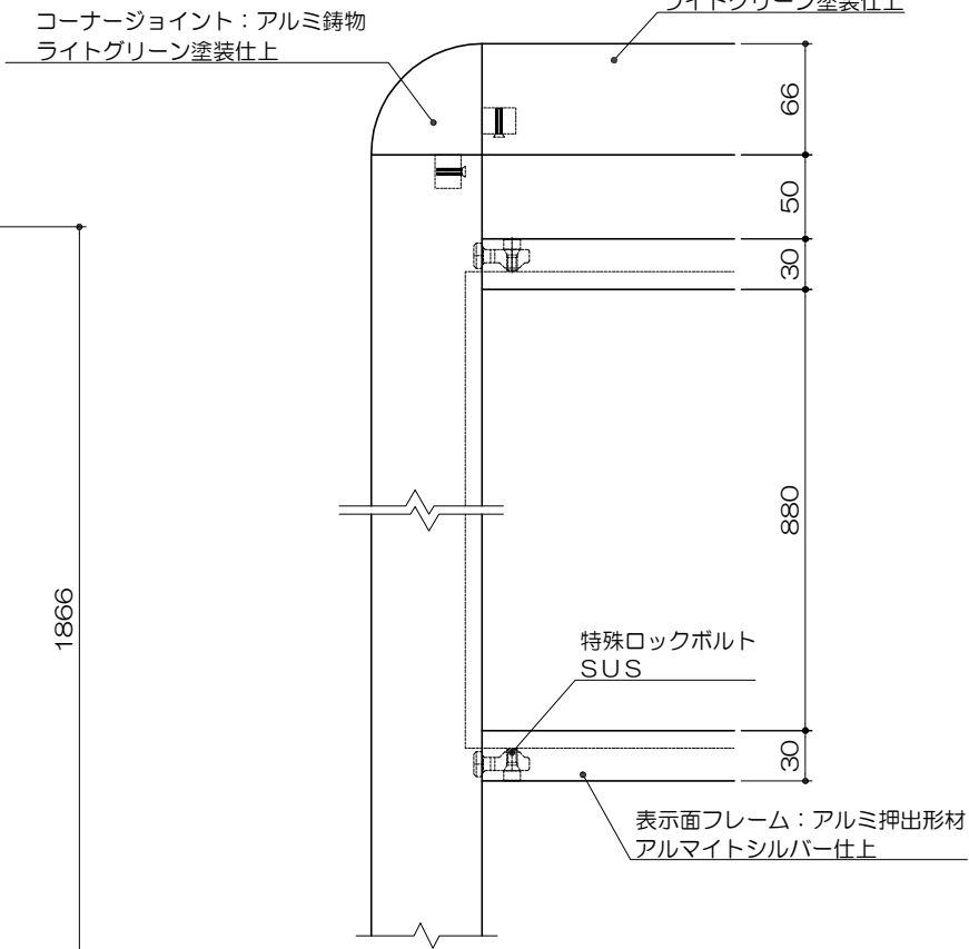
正面図 S= 1:5
