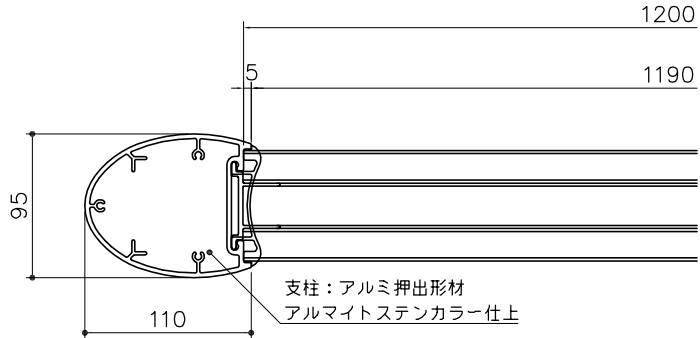
側面図 S= 1：20
