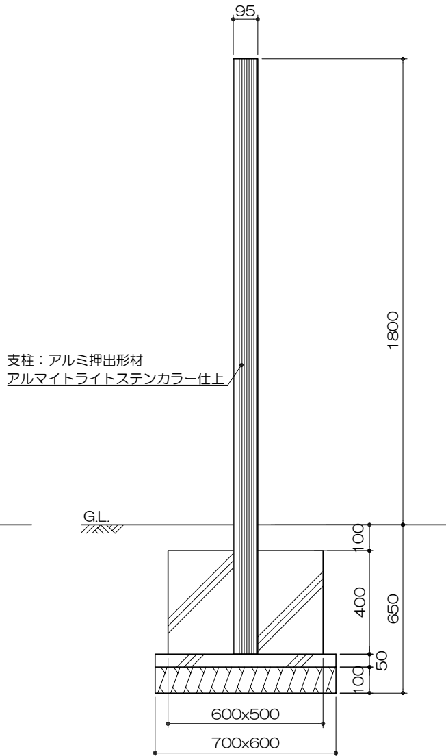
立面図 S= 1 : 5
