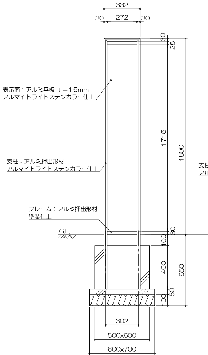
立面図 S= 1 : 20
