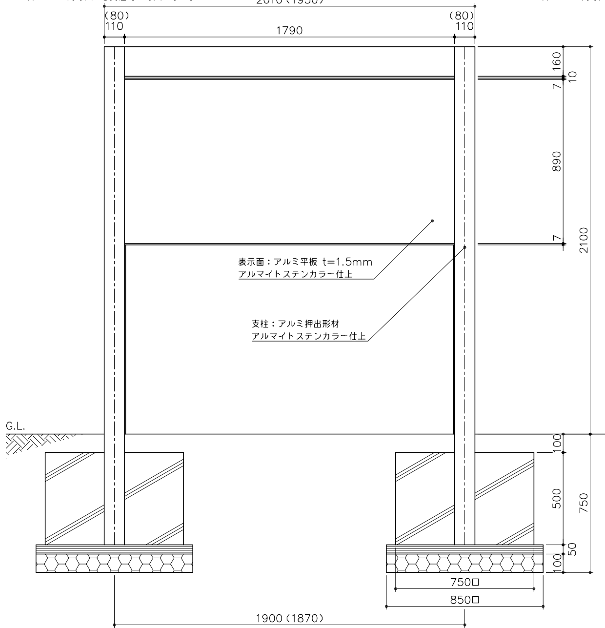
立面図 S= 1:20
