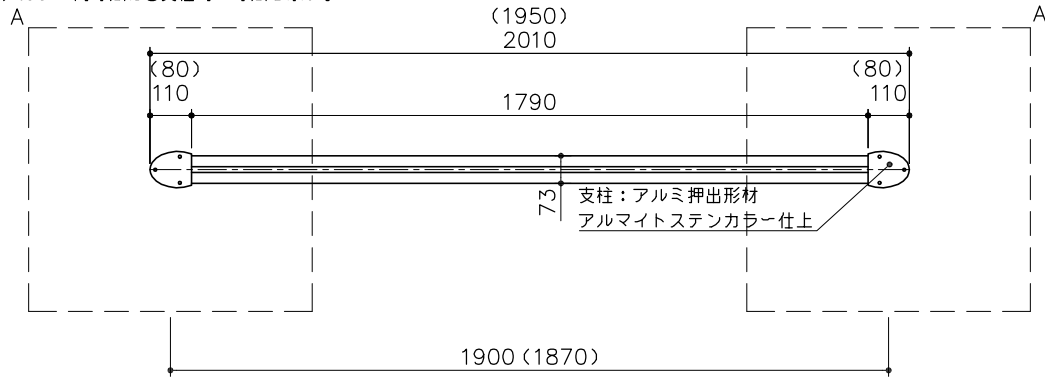
立面図 S= 1:20
