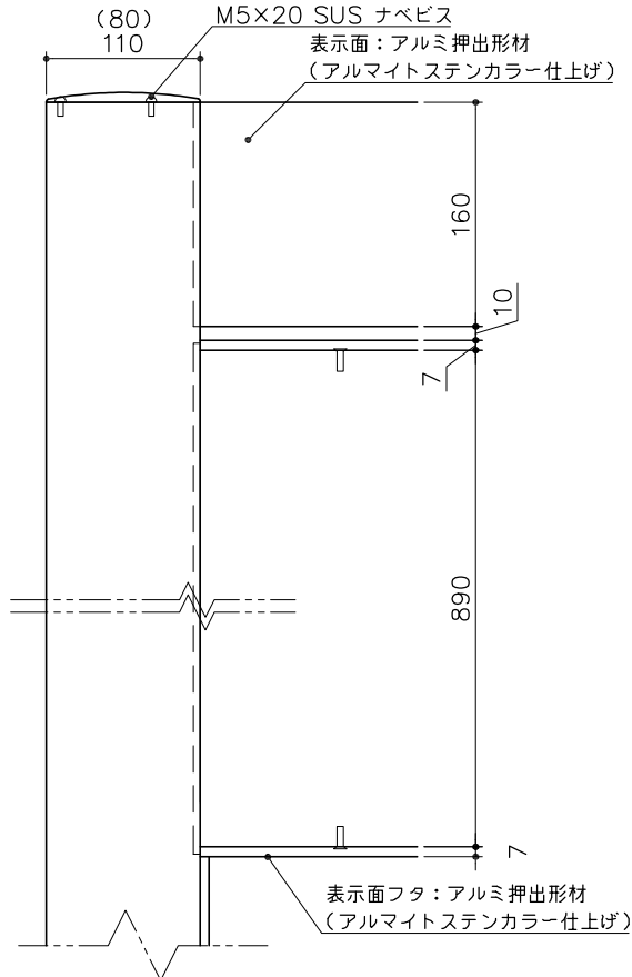
立面詳細図 S= 1:6
