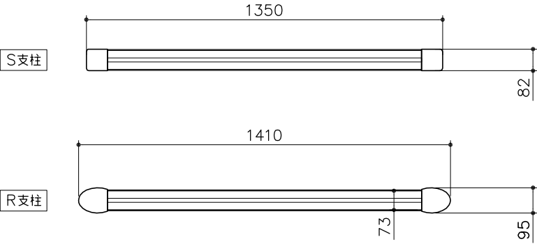
平面図 S= 1:20
