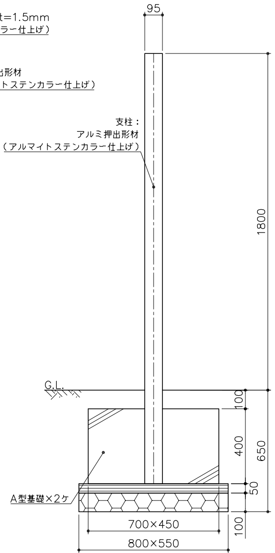
側面図 S= 1:20
