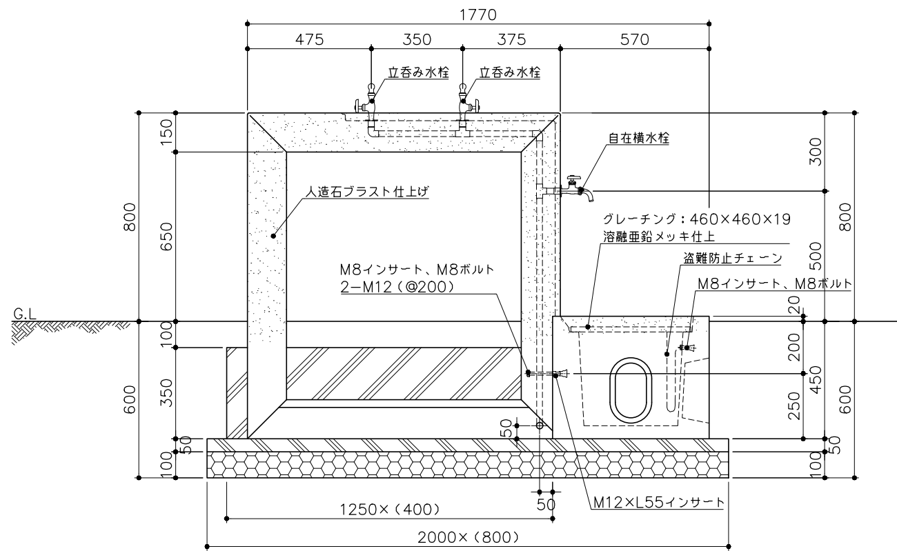
立面図 S= 1：20
