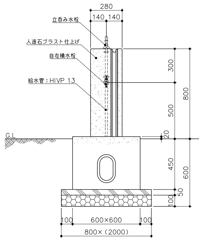
側面図 S= 1：20
