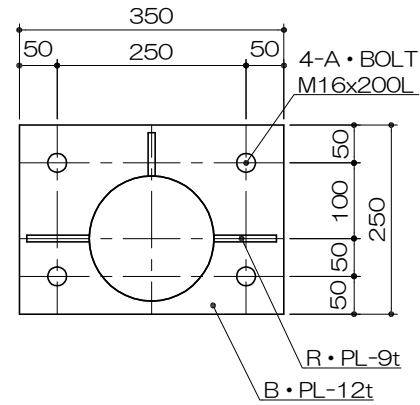
アンカープラン S= 1 : 10
