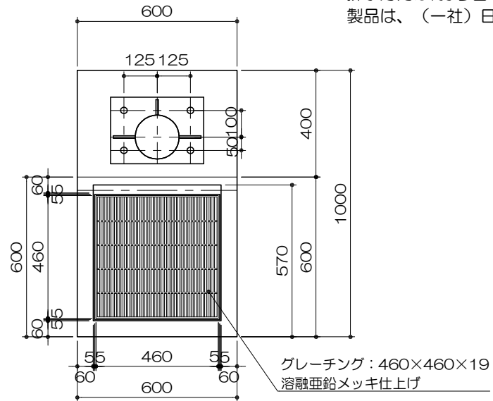
基礎平面図 S= 1 : 20
