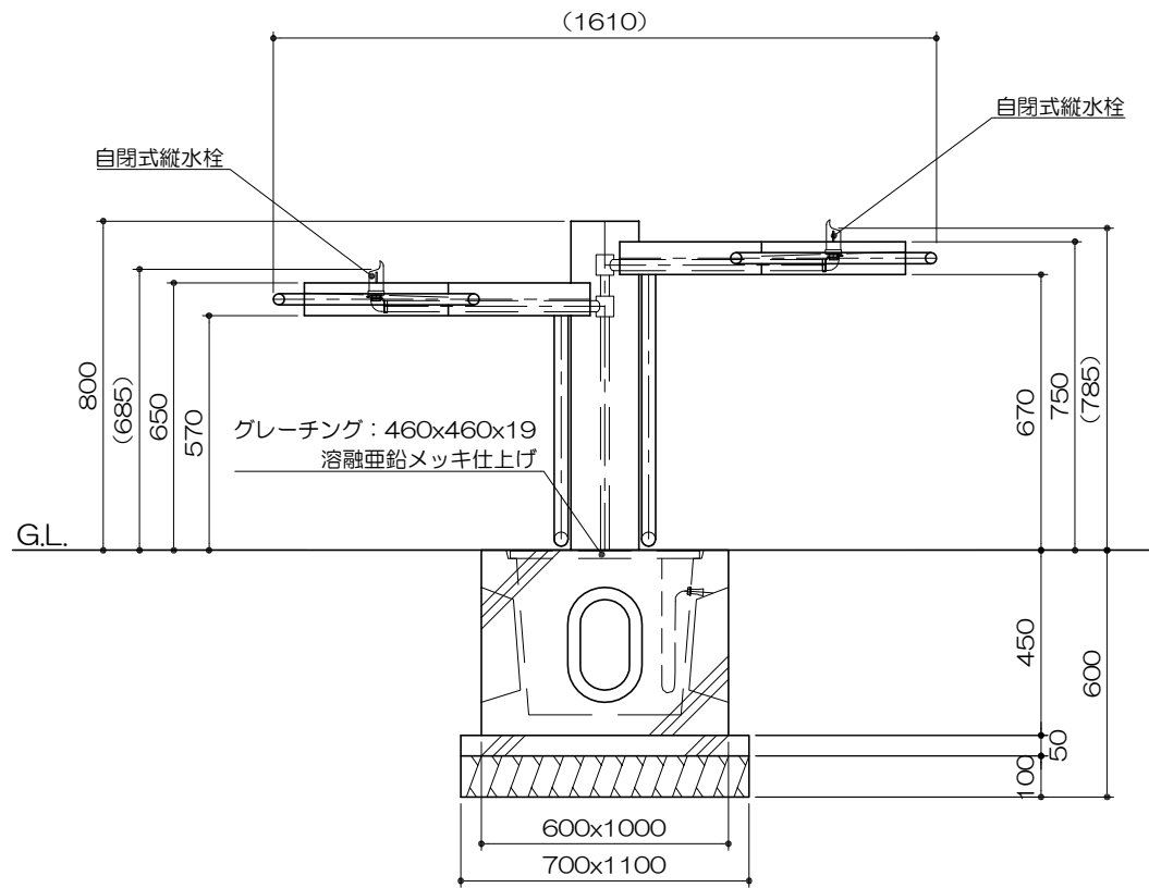
立面図 S= 1 : 20
