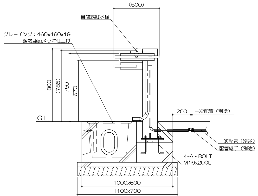
側面図 S= 1 : 20
