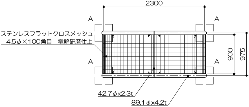
平面図 S= 1 : 50
