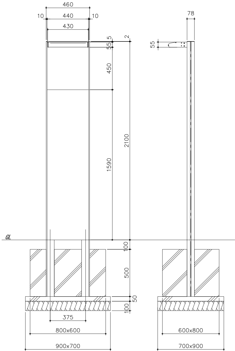
正面図 S= 1:20
