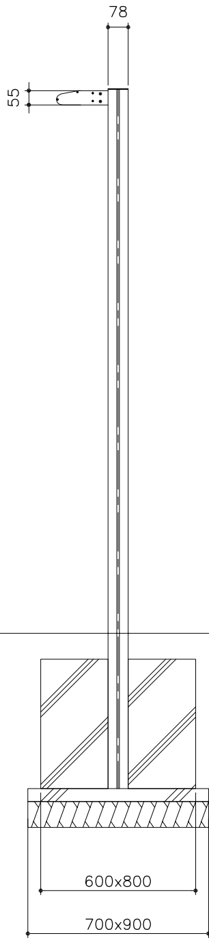
側面図 S= 1:20
