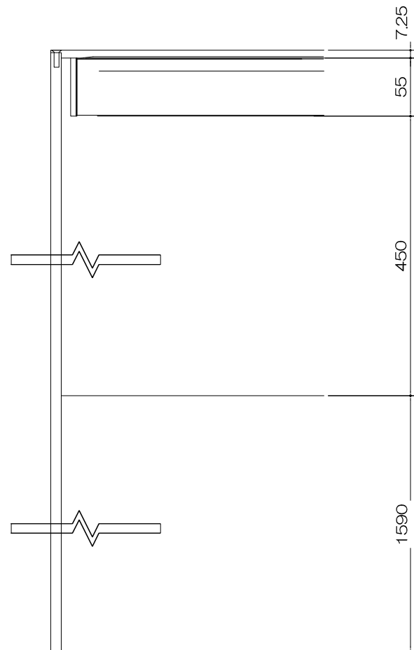
正面図 S= 1:5
