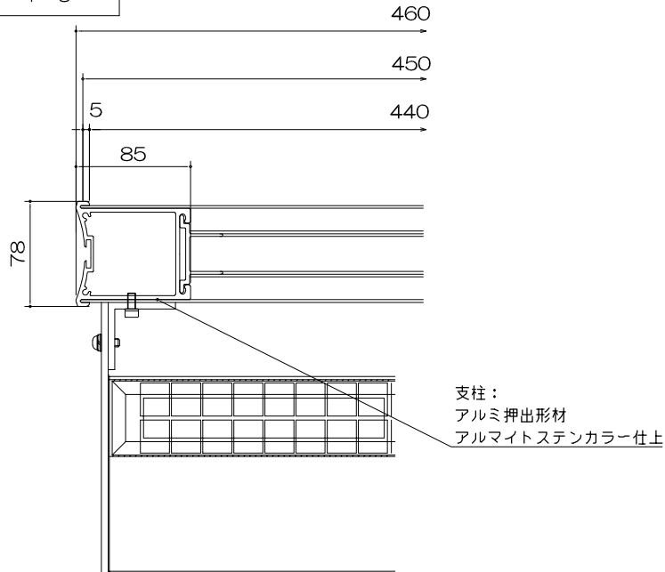
正面図 S= 1:5
