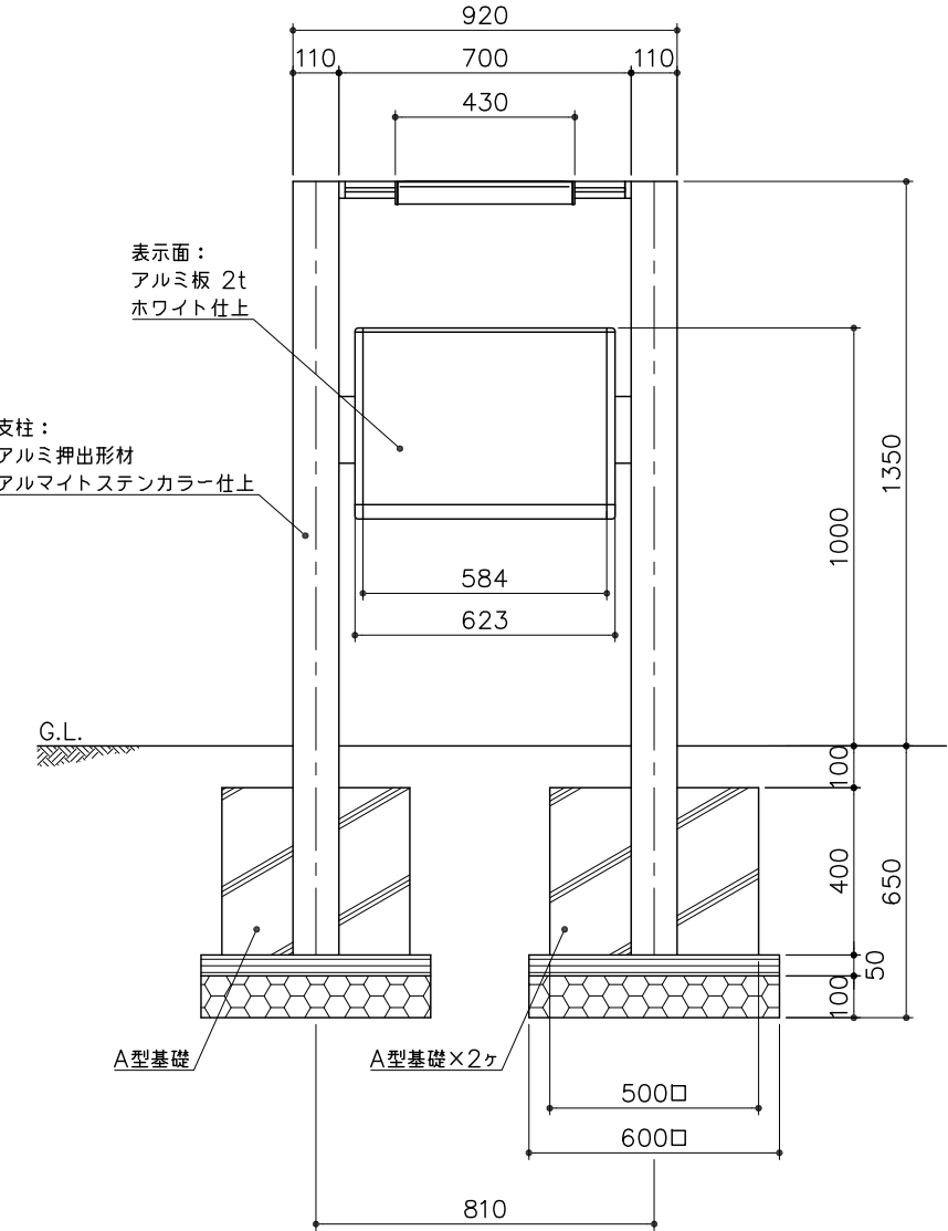
正面図 S= 1:20
