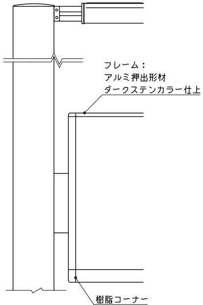
正面図 S= 1:10
