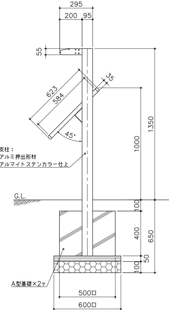
側面図 S= 1:20
