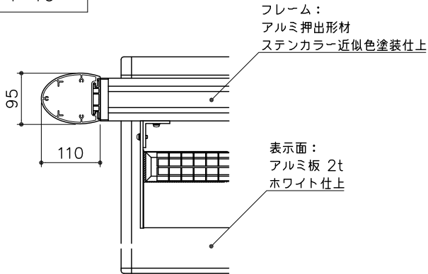
平面図 S= 1:10
