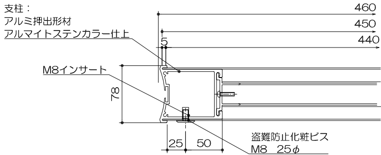
裏面図 S= 1:5
