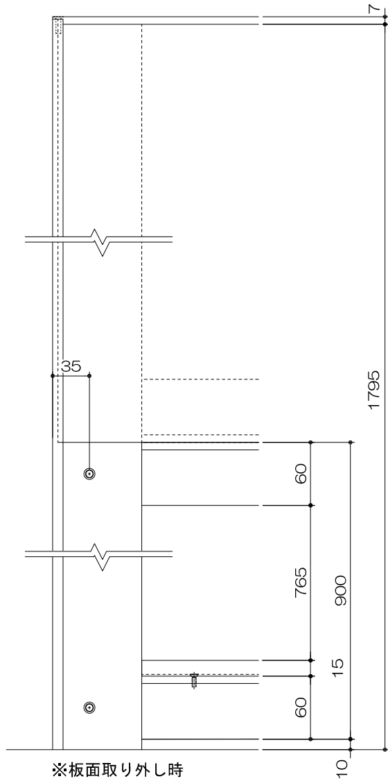
裏面図 S= 1:5
