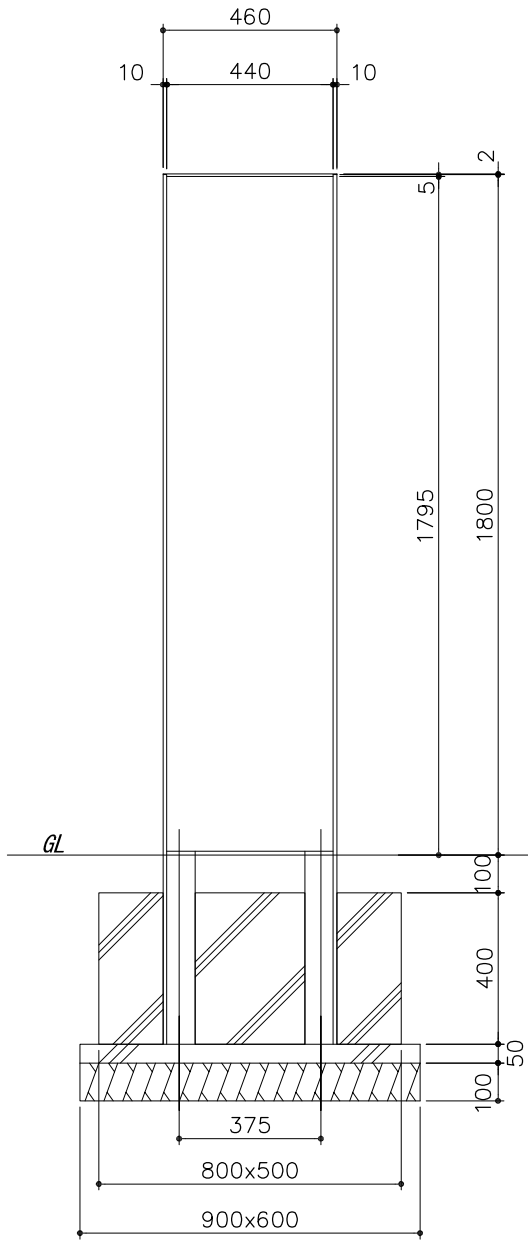
正面図 S= 1:20
