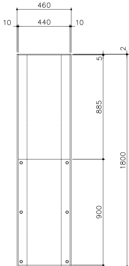
背面図 S= 1:20
