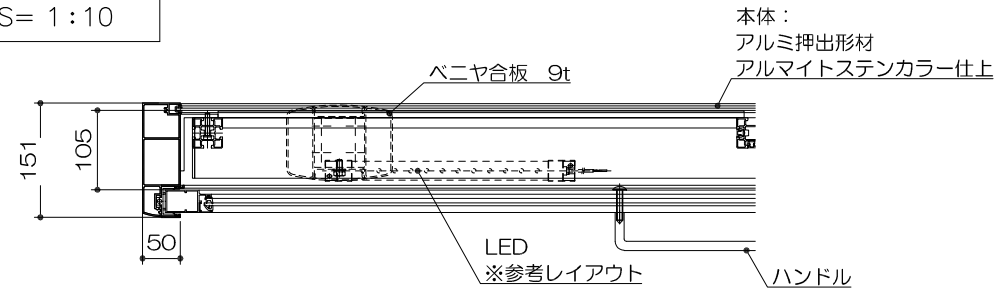
正面図 S= 1 : 10
