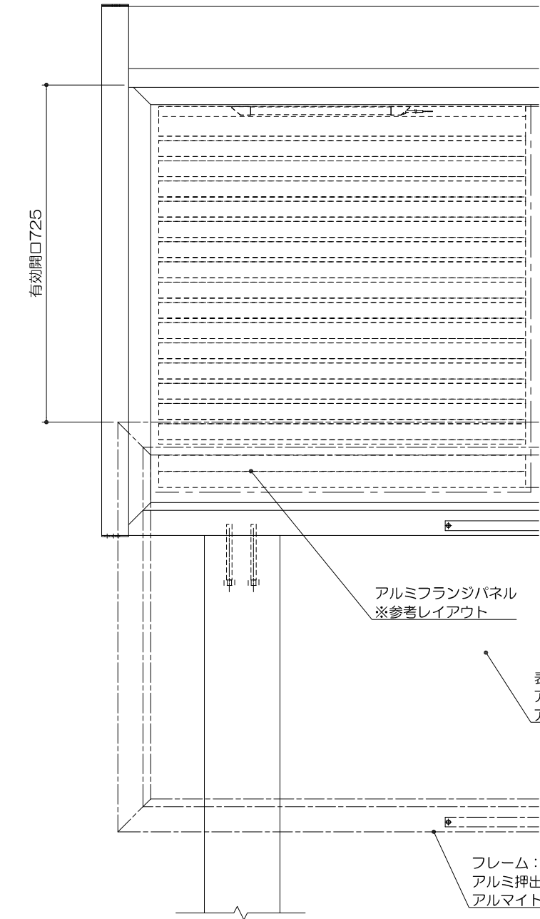
正面図 S= 1 : 10
