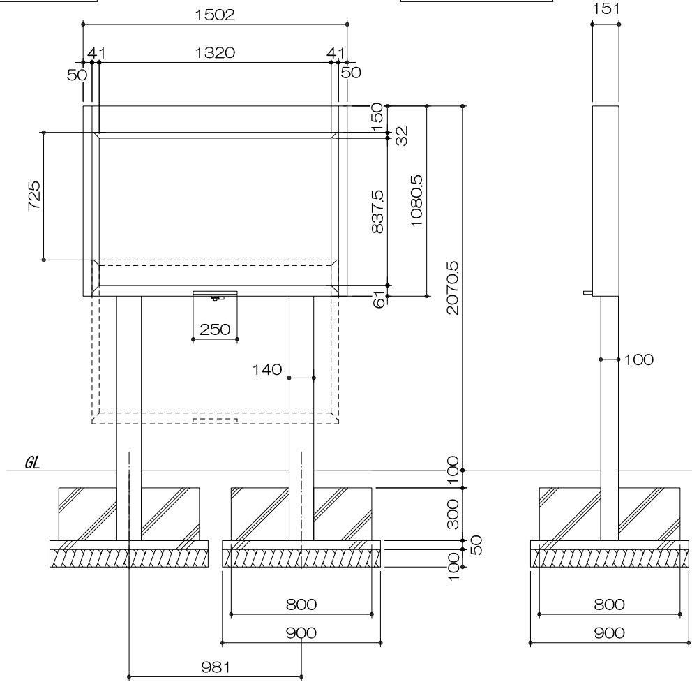
正面図 S= 1 : 30
