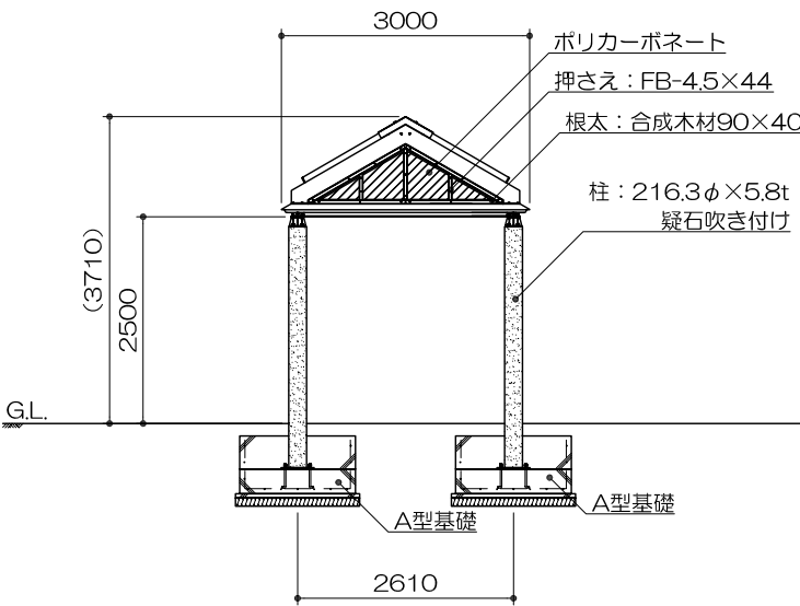
側面図 S= 1 : 100
