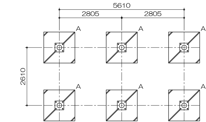
基礎平面図 S= 1 : 100
