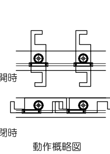
a部詳細図 S= 1 : 20
