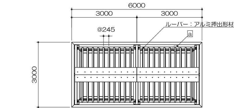
平面図 S= 1 : 100
