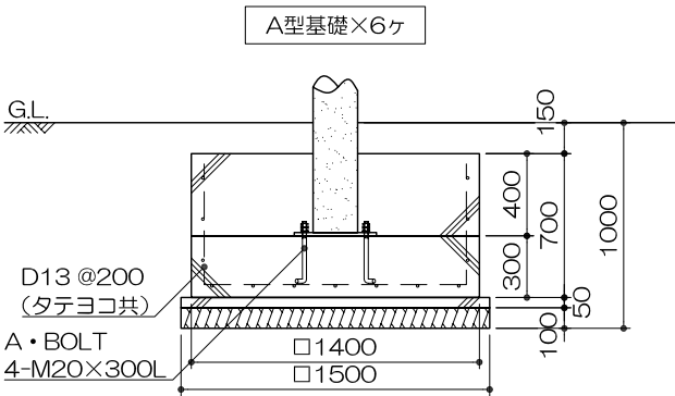
基礎リスト S= 1 : 40
