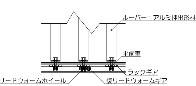
機能部分断面平面図 S= 1 : 20
