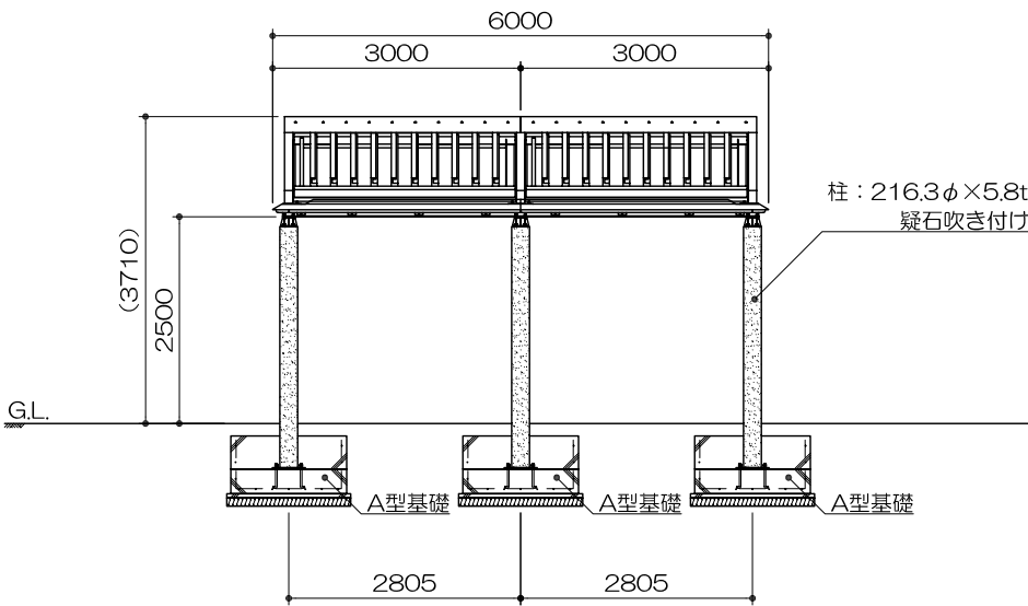
立面図 S= 1 : 100
