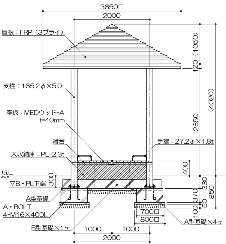
立面図 S= 1 : 60
