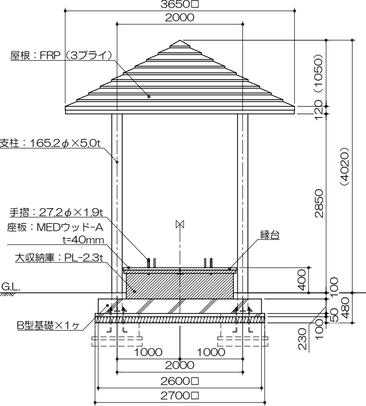
側面図 S= 1 : 60
