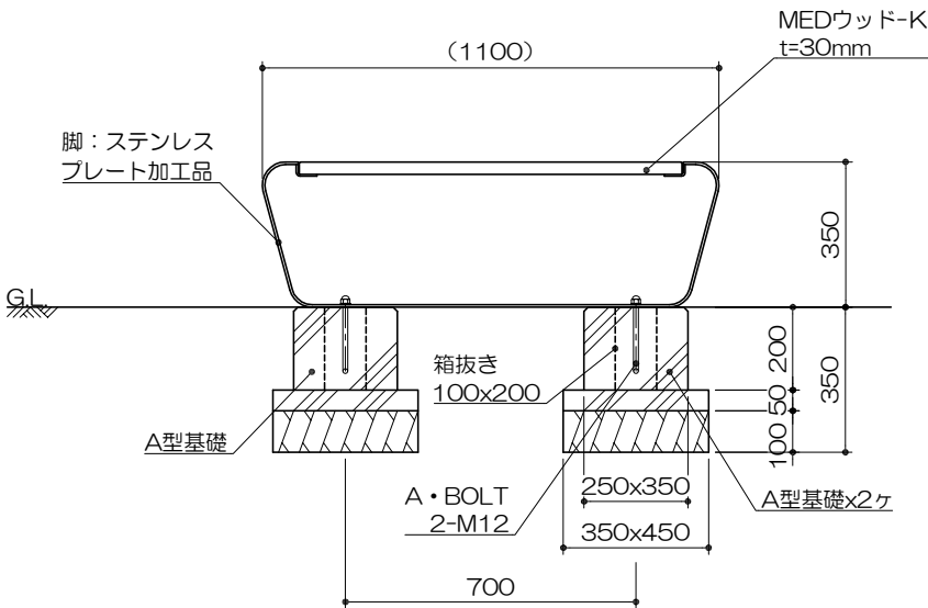
立面図 S= 1 : 20
