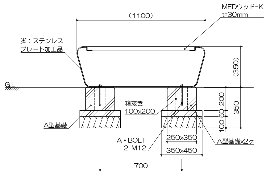
立面图 S= 1 : 20
