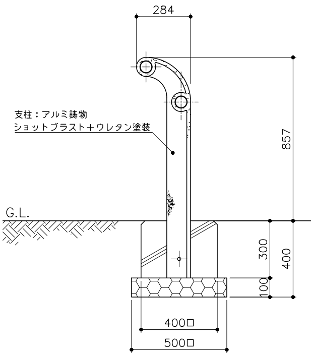
側面図 S= 1:20
