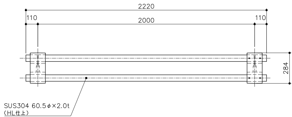
平面図 S= 1:20
