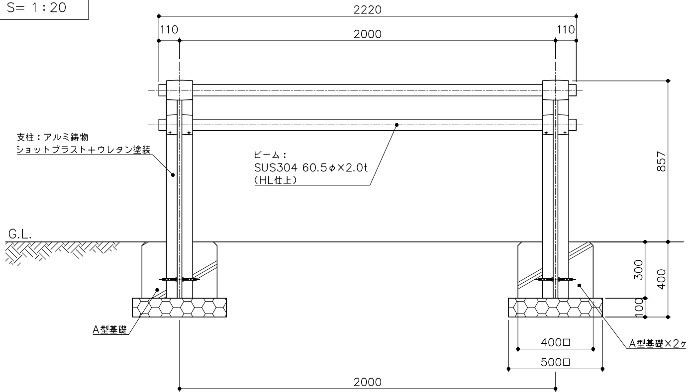
基礎平面図 S= 1:20
