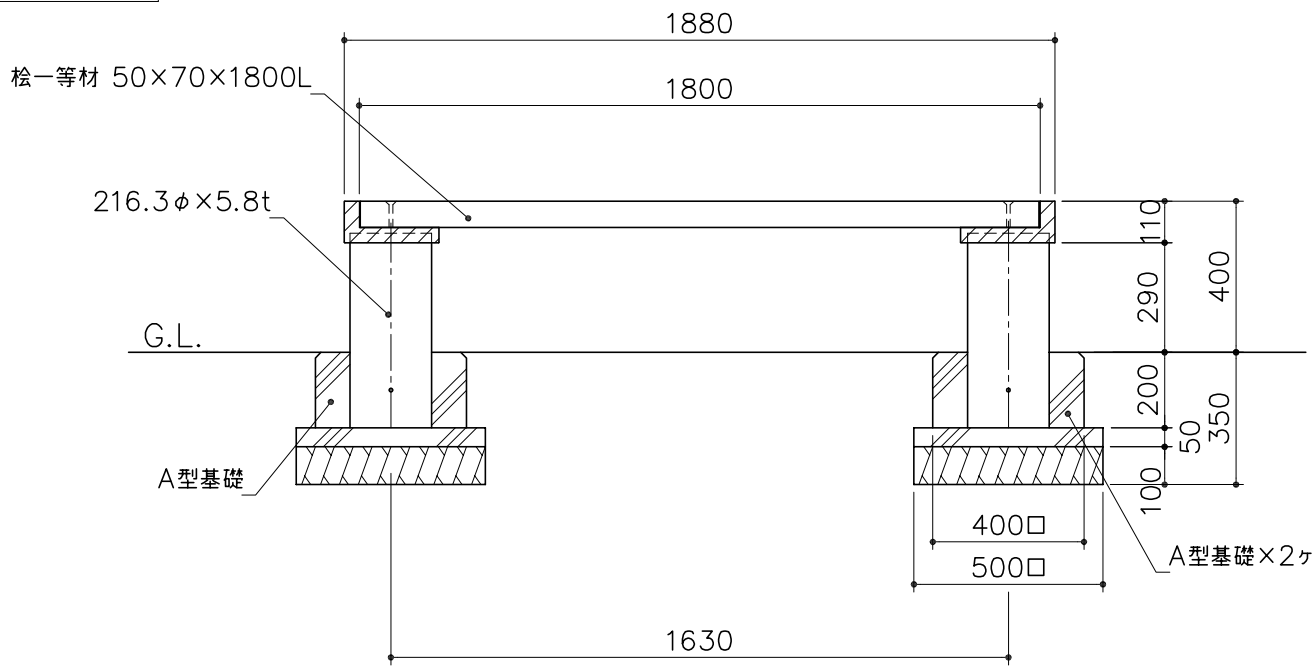
立面図 S= 1：20
