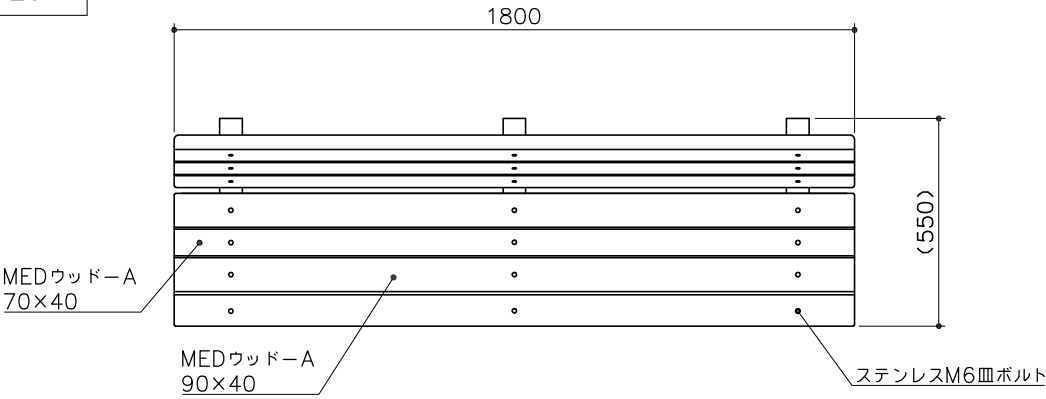
平面図 S= 1 : 20
