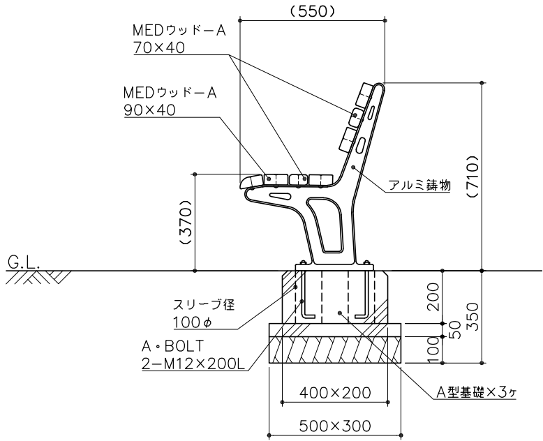
側面図 S= 1 : 20
