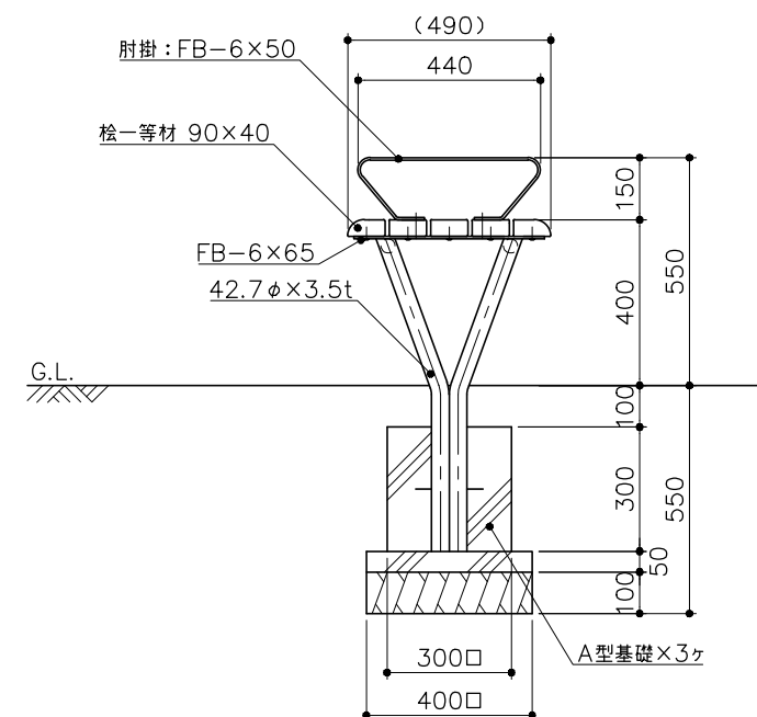
側面図 S= 1 : 20
