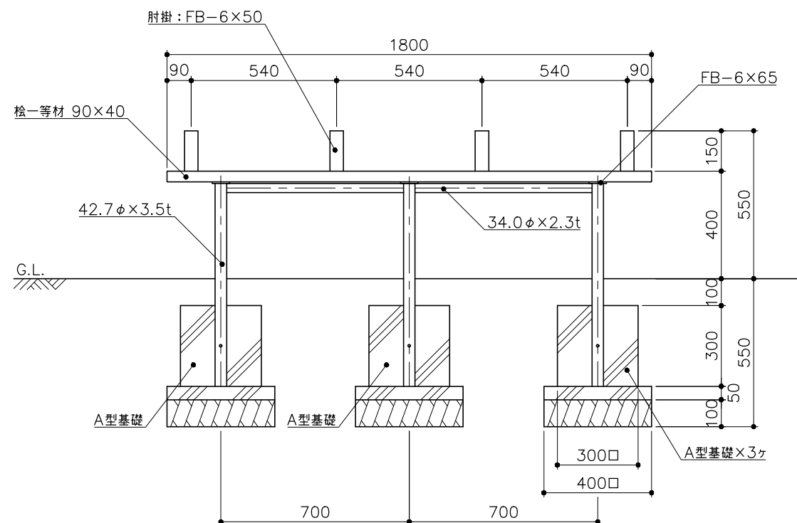
立面図 S= 1 : 20
