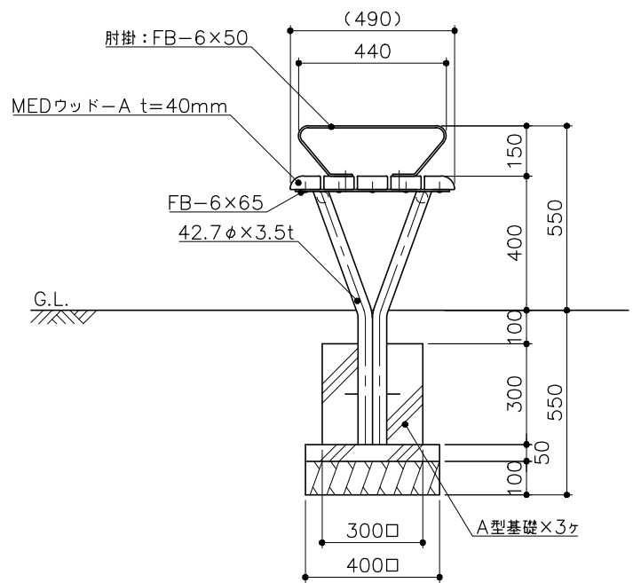
側面図 S= 1 : 20
