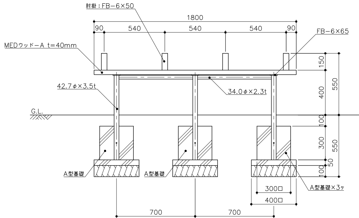
立面図 S= 1 : 20
