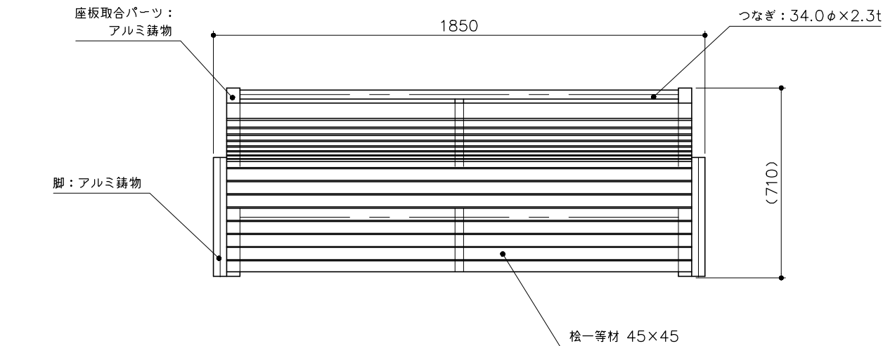
平面図 S= 1 : 20
