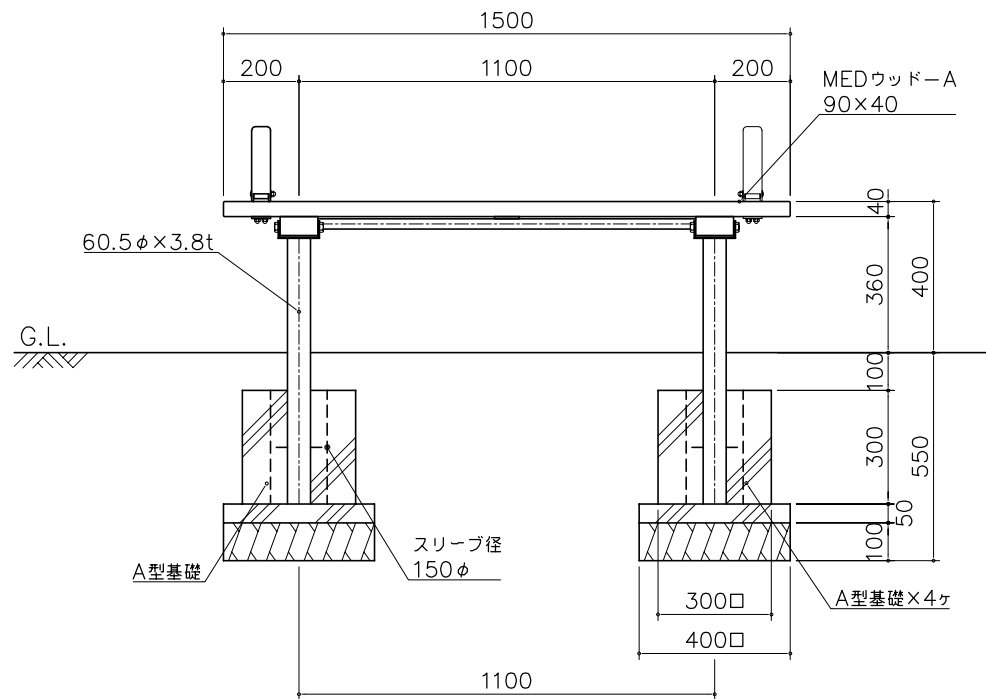
立面図 S= 1:20
