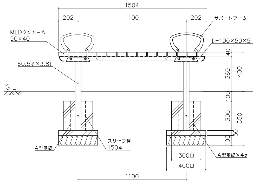
側面図 S= 1:20
