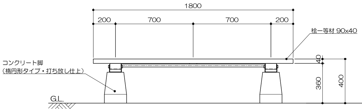
立面図 S= 1 : 20
