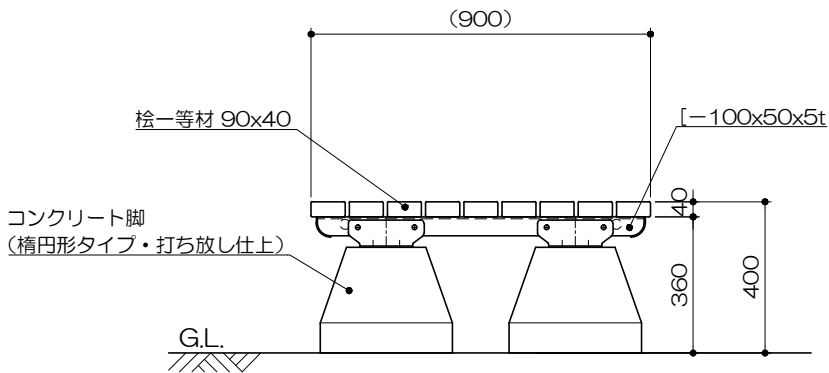
側面図 S= 1 : 20
