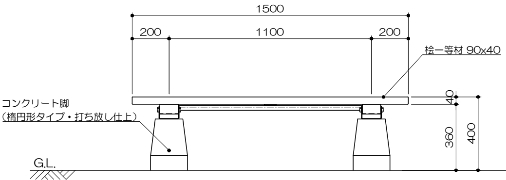
立面図 S= 1 : 20
