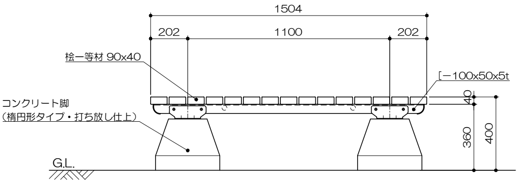
側面図 S= 1 : 20
