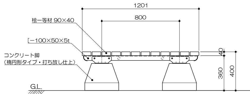
側面図 S= 1 : 20
