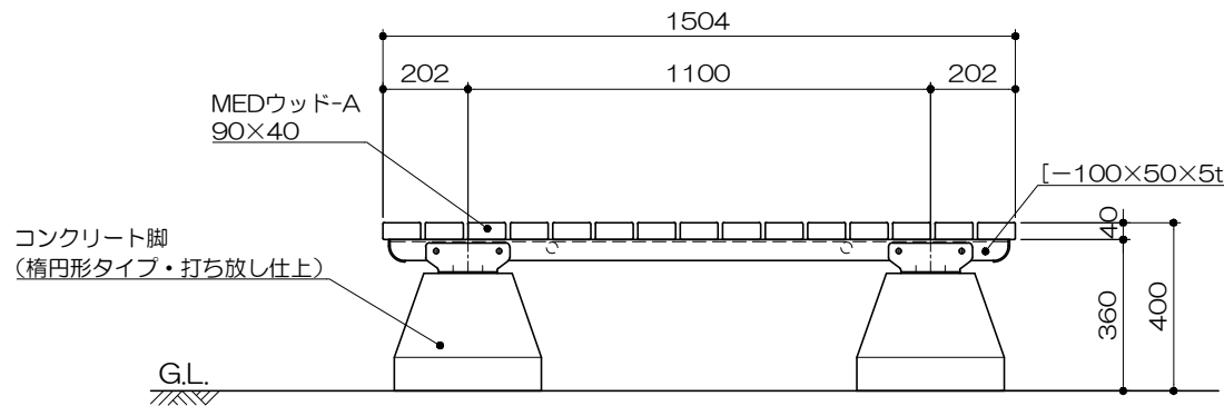
側面図 S= 1 : 20
