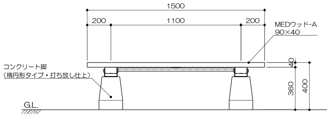
立面図 S= 1 : 20
