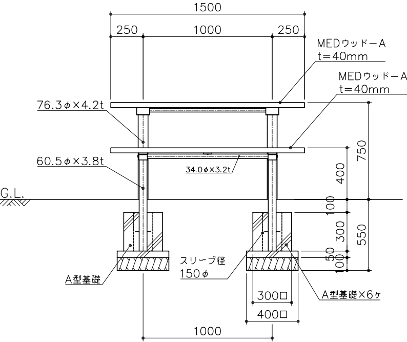
立面図 S= 1:30
