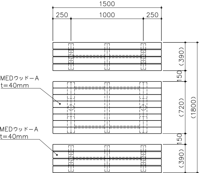
平面図 S= 1:30
