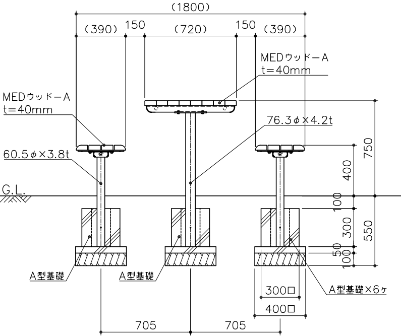
側面図 S= 1:30
