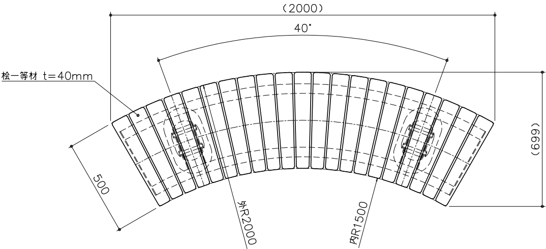
平面図 S= 1：20
