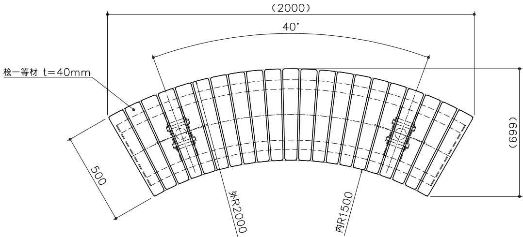
平面図 S= 1：20
