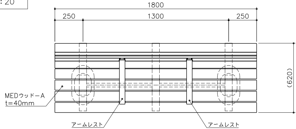
基礎平面図 S= 1 : 20
