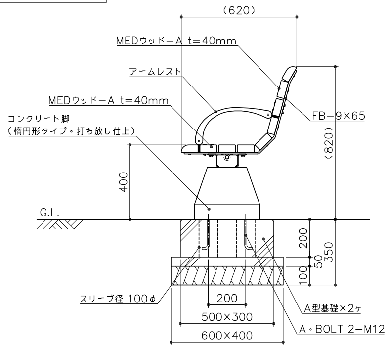
側面図 S= 1 : 20
