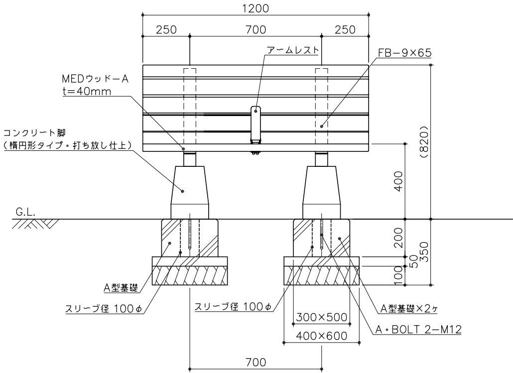
立面図 S= 1 : 20
