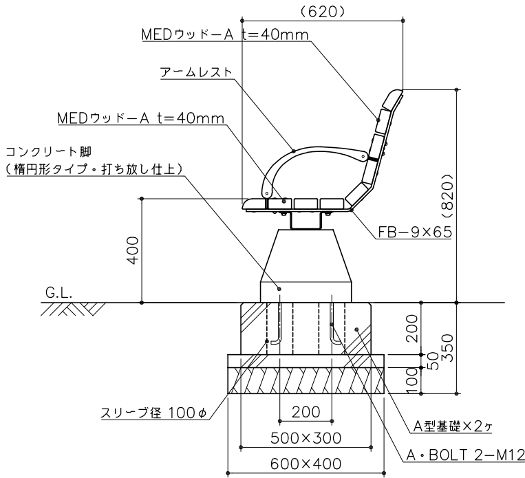
側面図 S= 1 : 20
