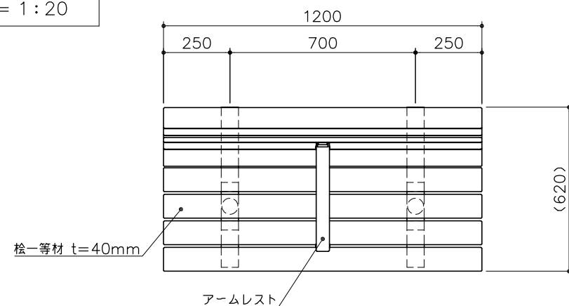
基礎平面図 S= 1 : 20
