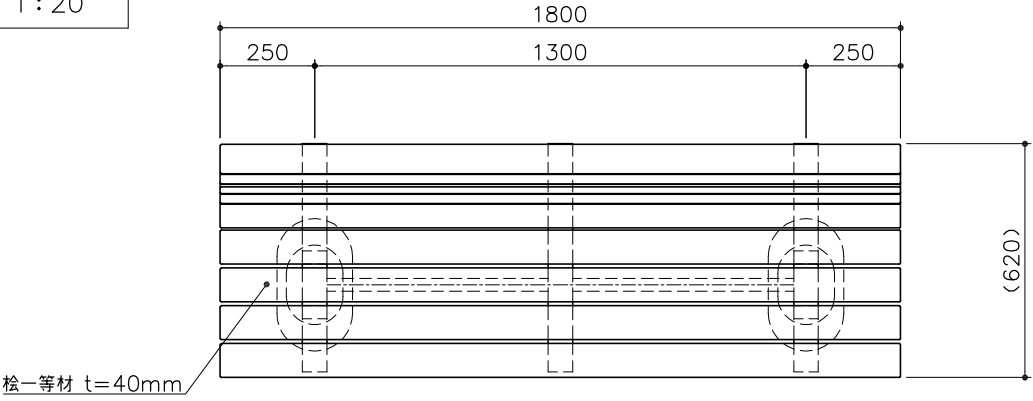
平面図 S= 1 : 20
