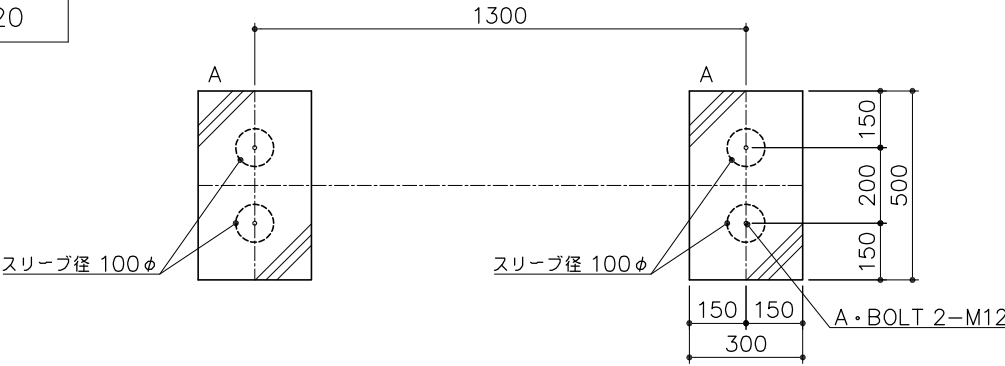
立面図 S= 1 : 20
