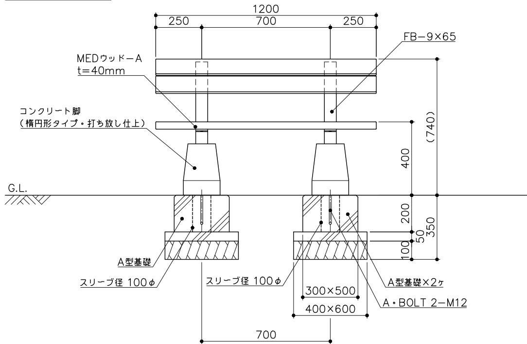
立面図 S= 1:20
