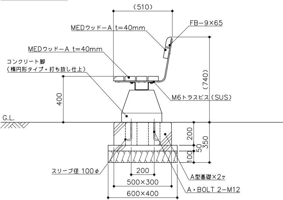
側面図 S= 1:20
